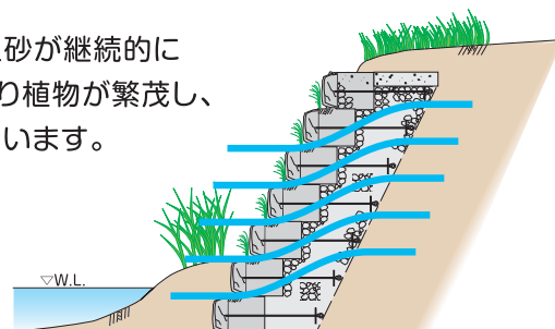
護岸の透水性を確保
